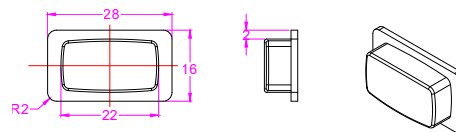
Key cap
